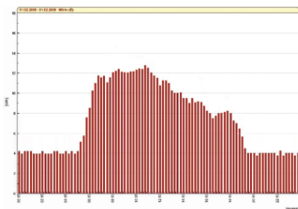
Lastgang nach Optimierung
